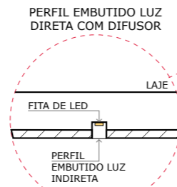
DETALHE esc.1:20 cotas em centímetros
